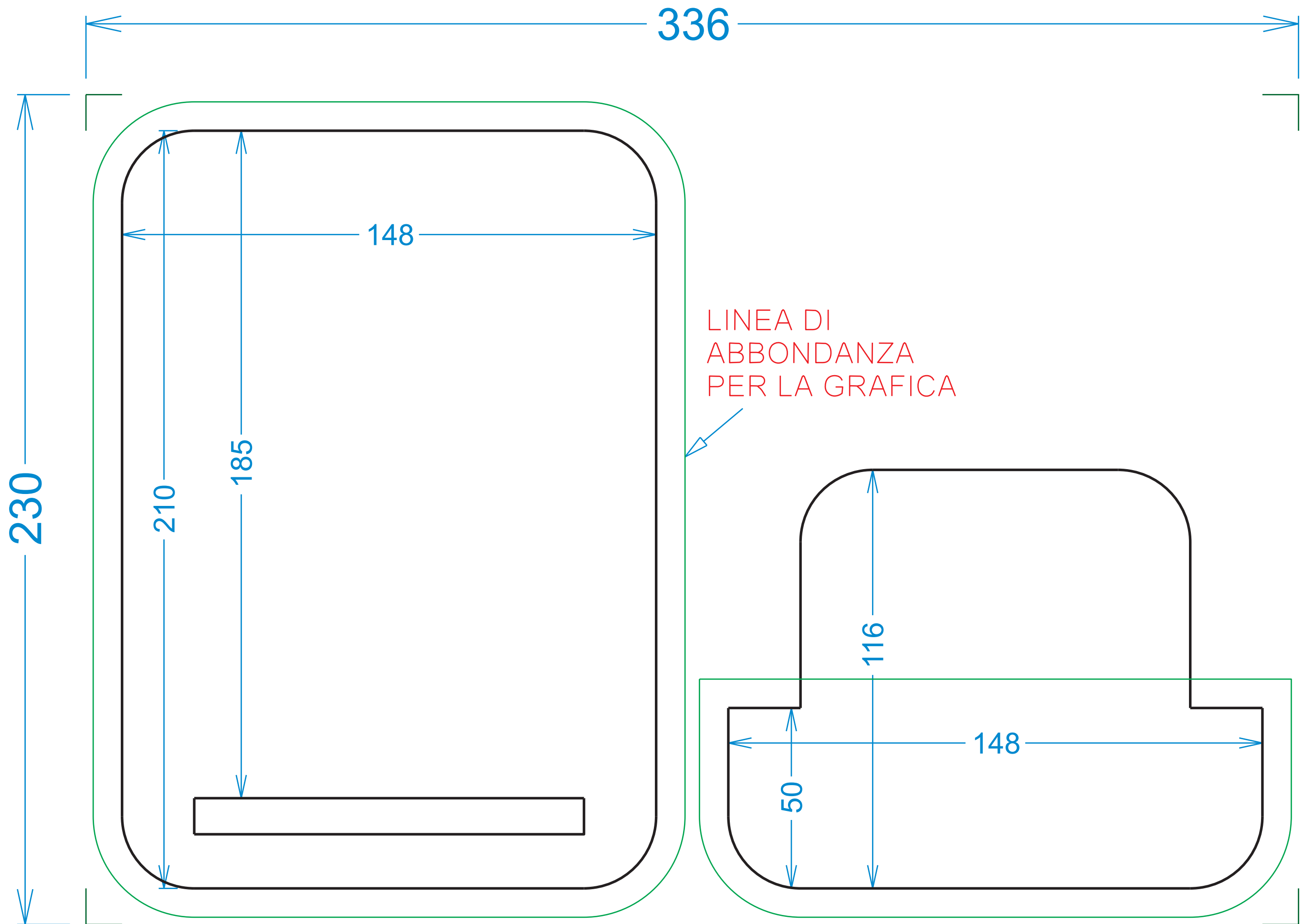
PINZA LATO STAMPA COD. 800_3107-02_DIS1
