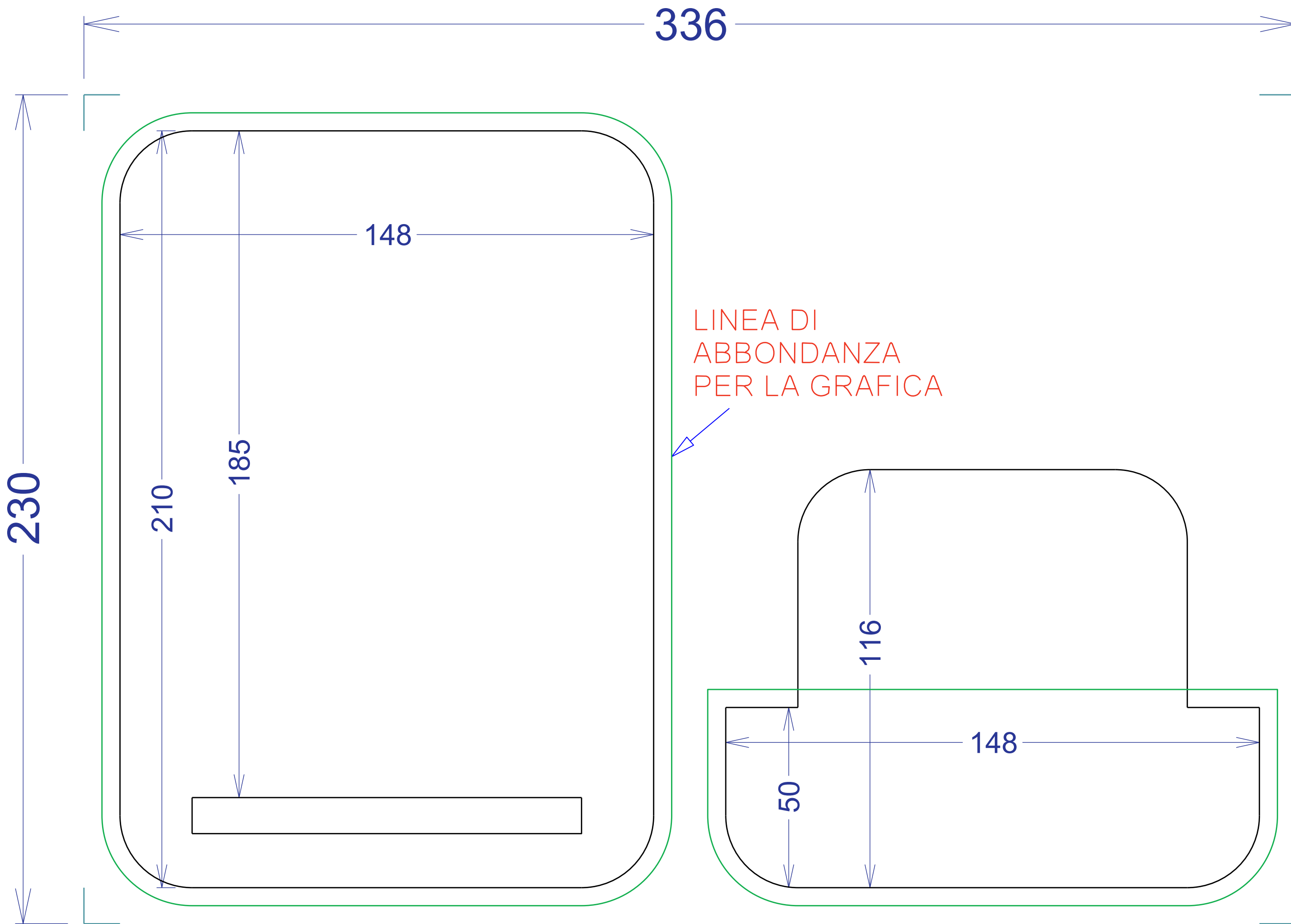
PINZA LATO STAMPA COD. 800_3107-02_DIS1
